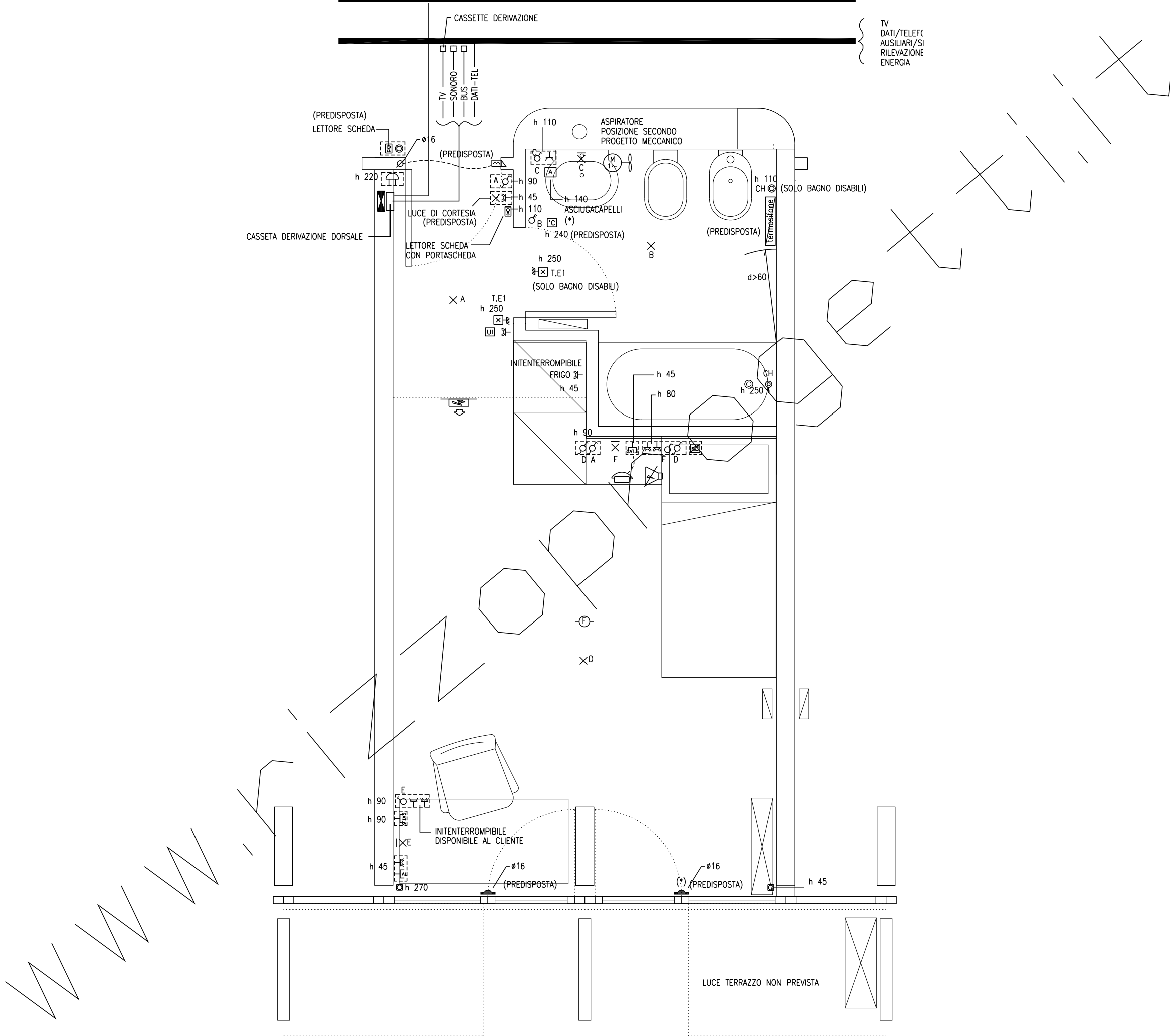
CAMERA SINGOLA TIPO 15 unità al piano terra e 13 unità al piano primo di cui 1 attrezzata per disabili
